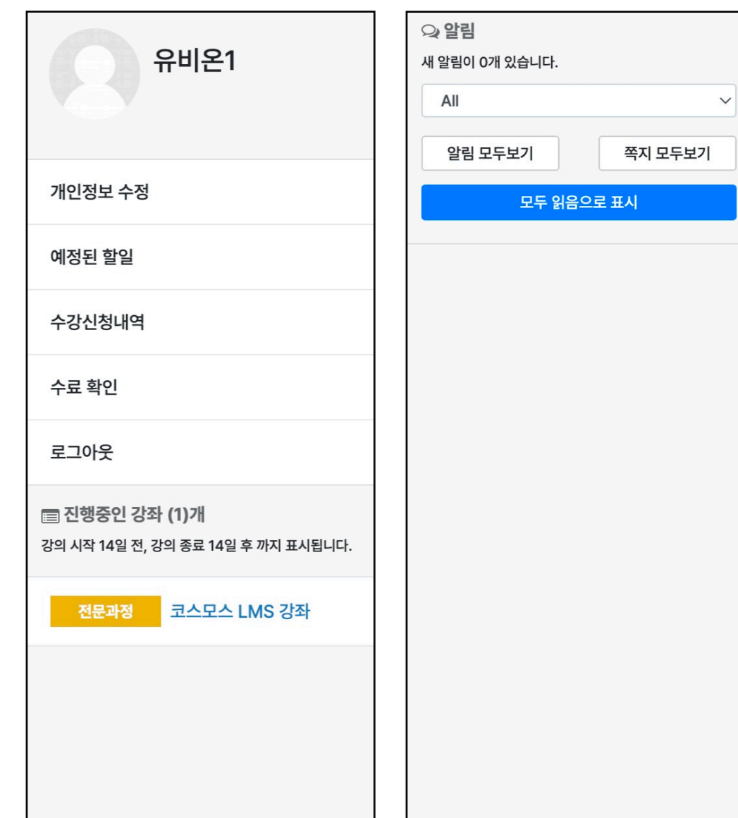
[개인 메뉴]
